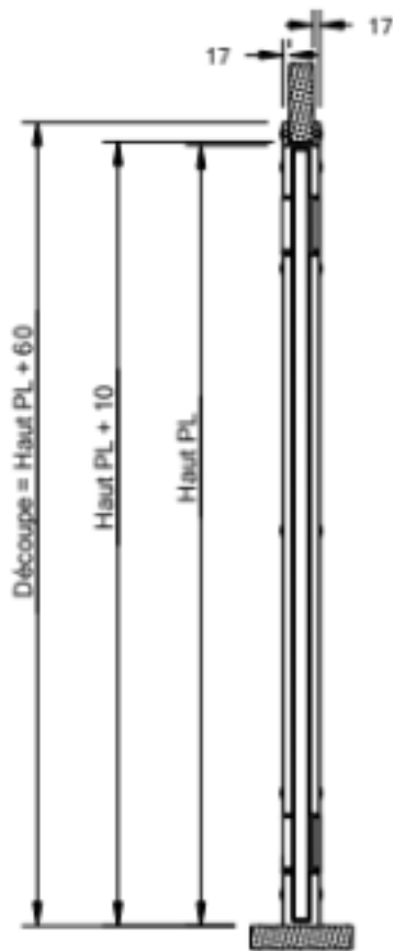
Coupe B-B
