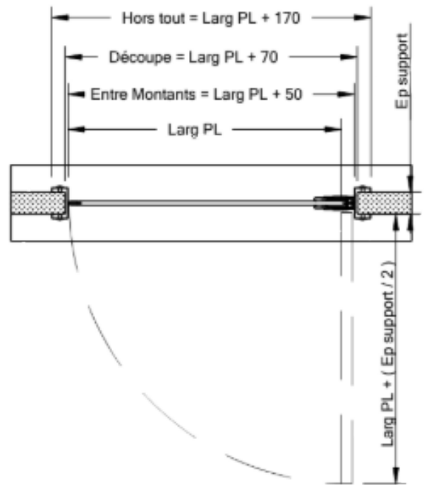
Coupe A-A
