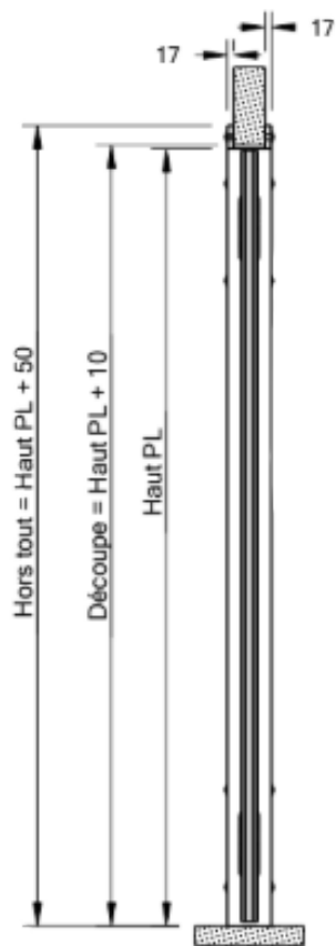
Coupe B-B
