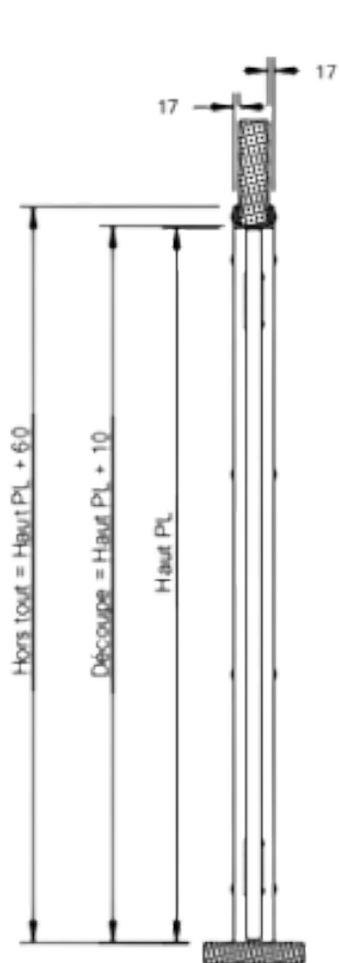
Coupe B-B
