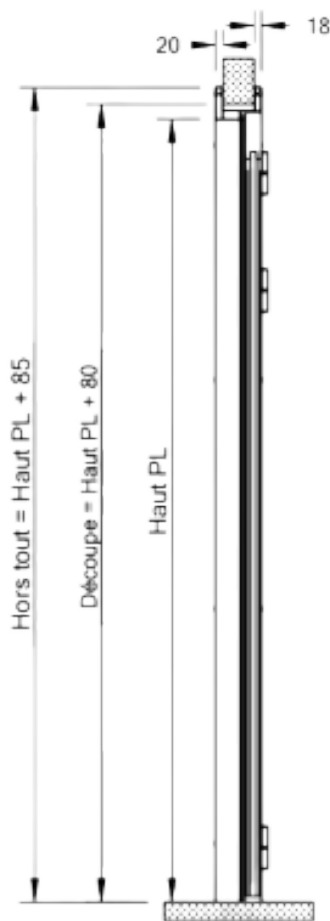
Coupe B-B
