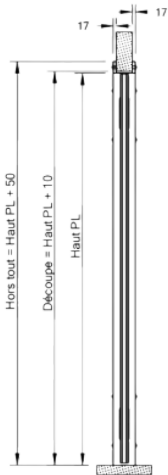
Coupe B-B
