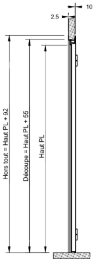
Coupe B-B
