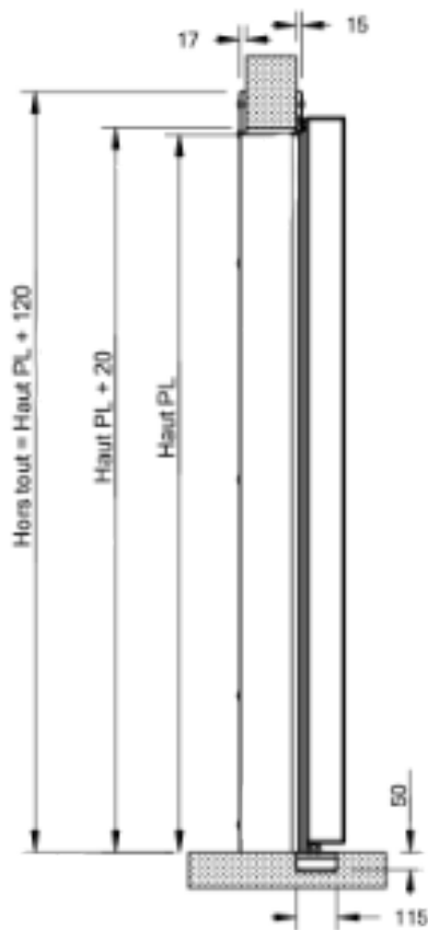
Coupe B-B
