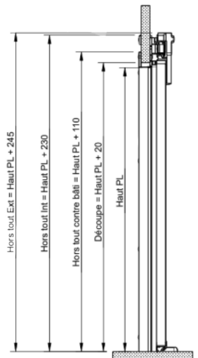
Coupe C-C
