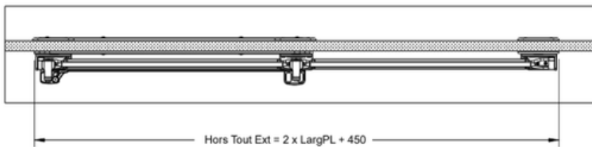
Coupe B-B
