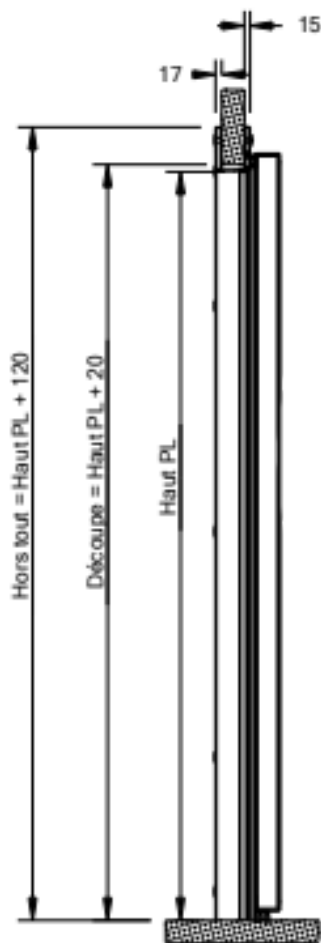
Coupe B-B
