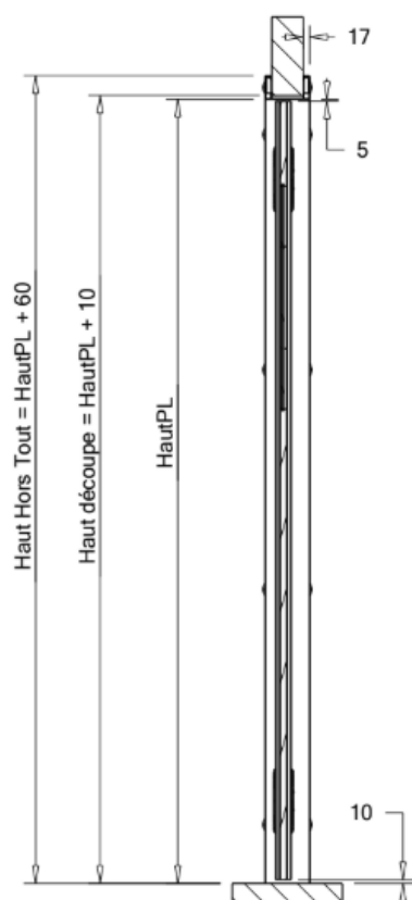
Coupe B-B
