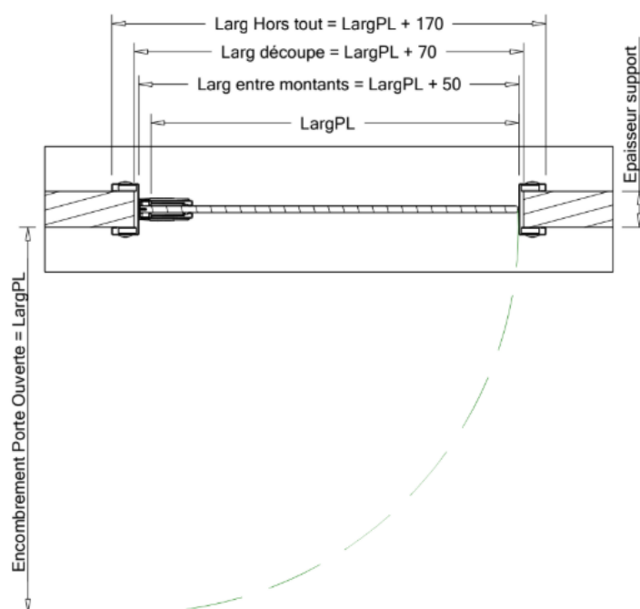
Coupe A-A
