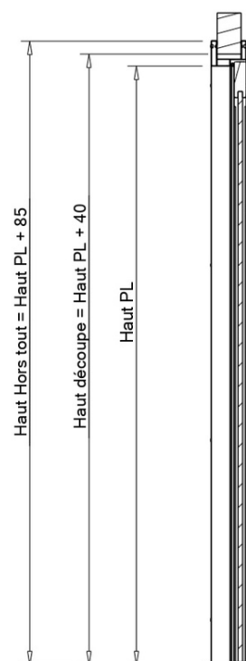
Coupe B-B
