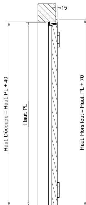
Coupe C-C
