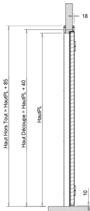
Coupe B-B
