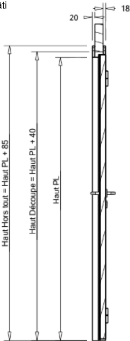
Coupe B-B
