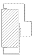
Profil Bâti / Contre-bâti
