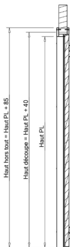
Coupe B-B
