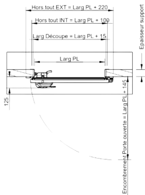
Coupe A-A
