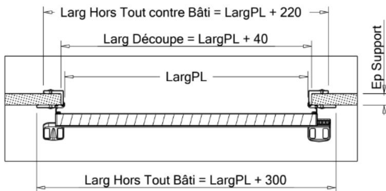
Coupe A-A
