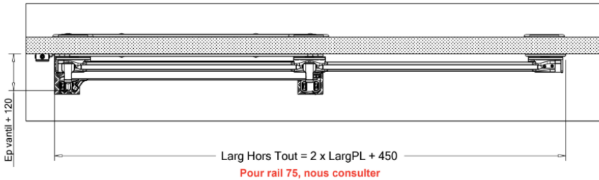
Coupe B-B
