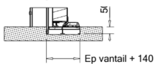
Coupe D-D
