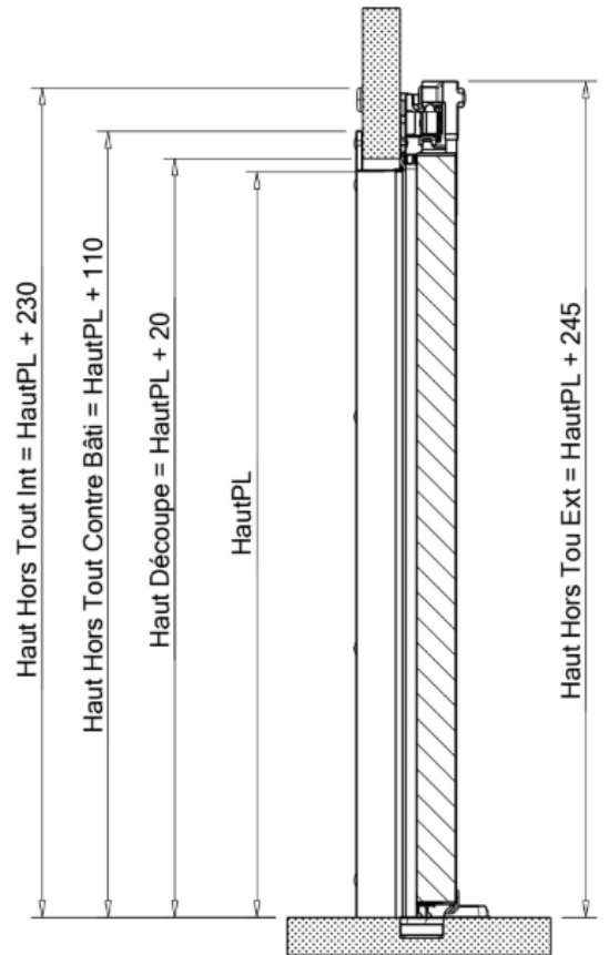
Coupe C-C
