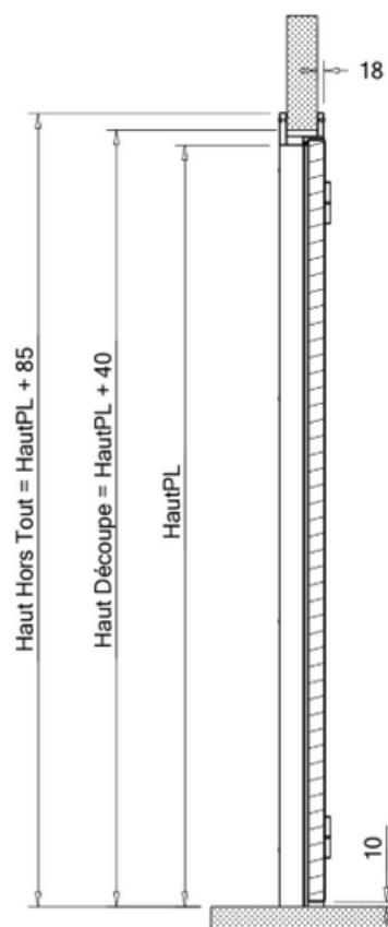
Coupe B-B
