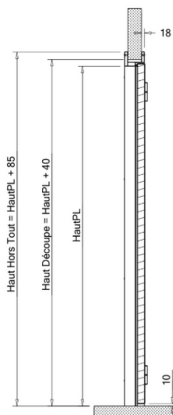
Coupe B-B
