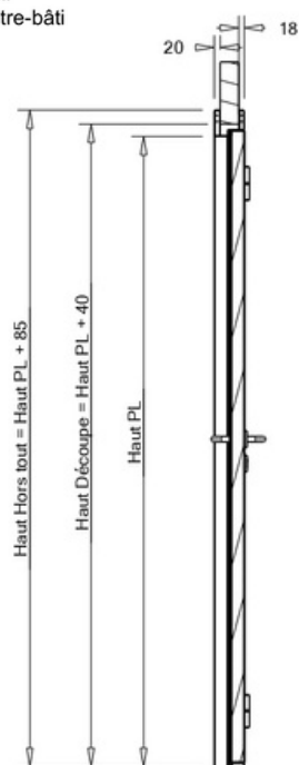
Profil Bâti / Contre-bâti
