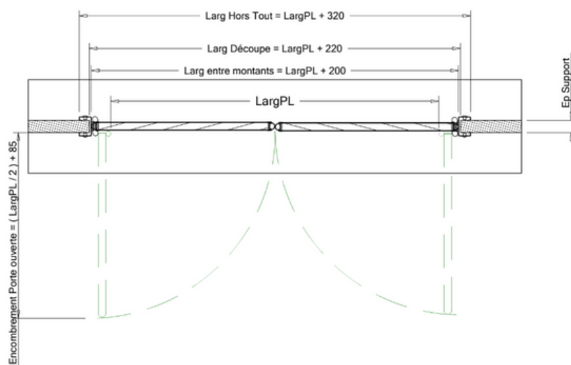
Coupe A - A
