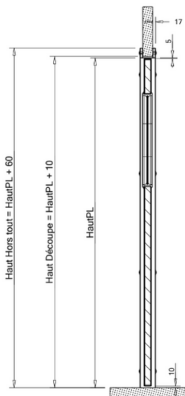
Coupe B-B
