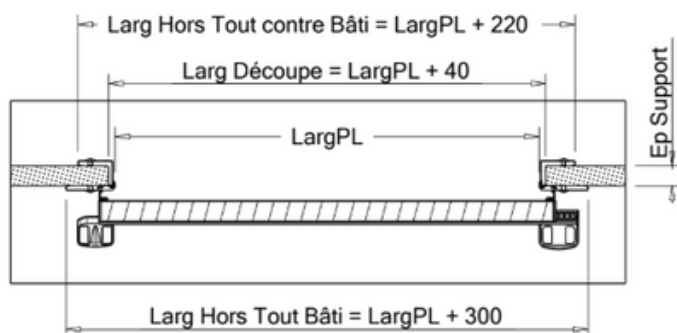
Coupe A-A
