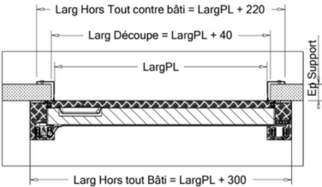
Coupe A-A
