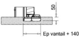
Coupe D-D
