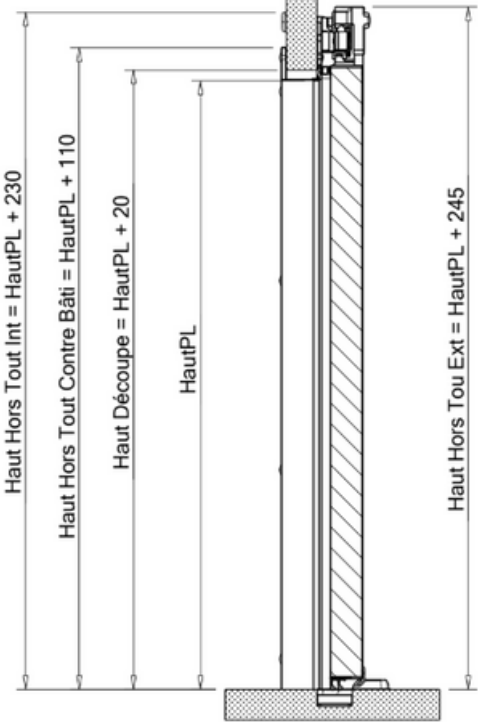
Coupe C-C
