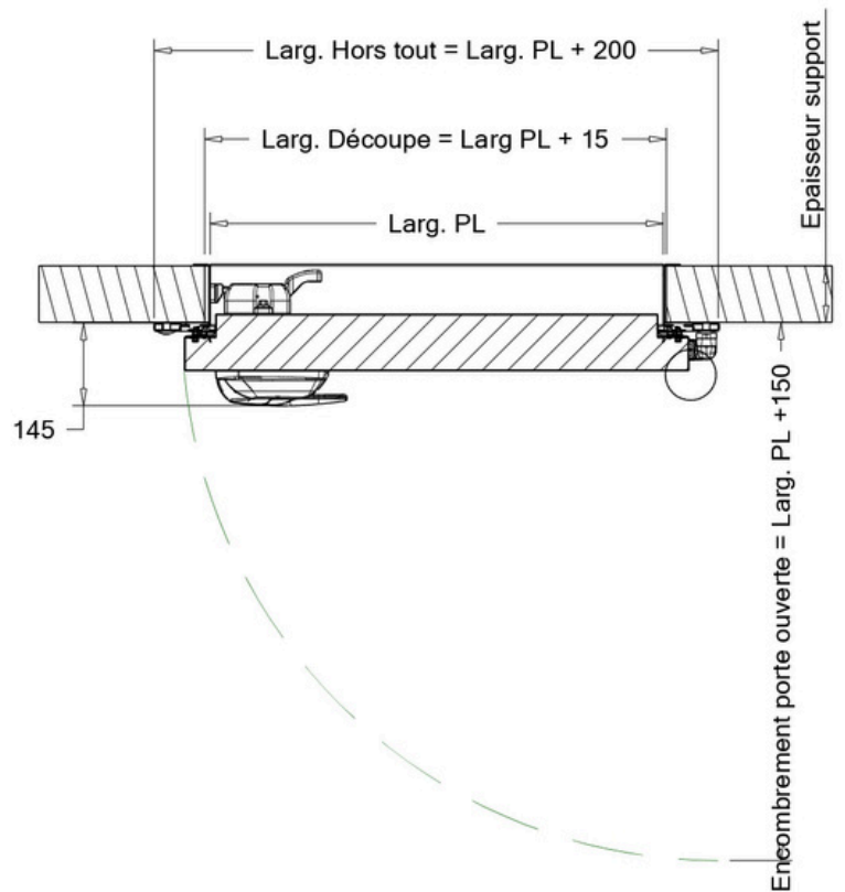
Coupe A-A
