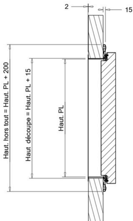
Coupe B-B
