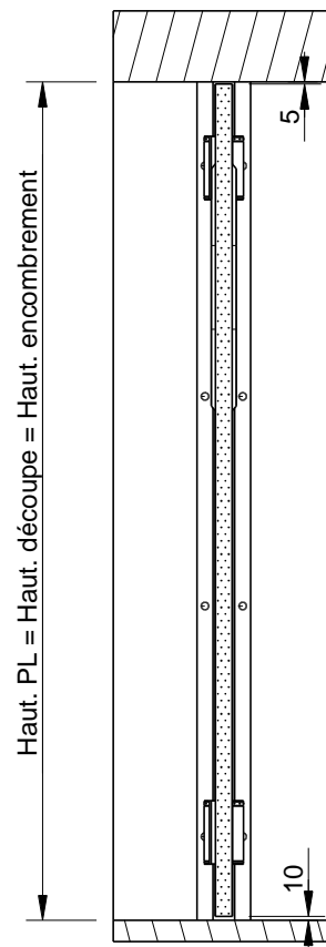
Coupe B-B
