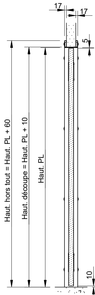
Coupe B-B
