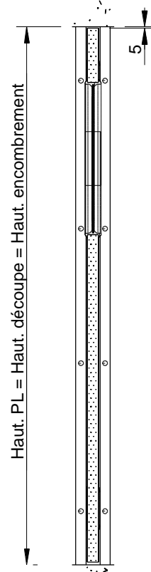
Coupe B-B
