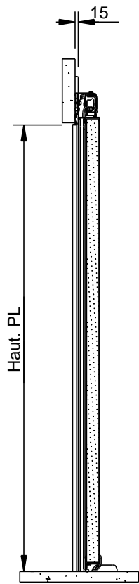
Coupe B-B
