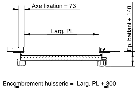
Coupe A-A
