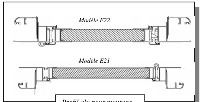
Profil alu pour montage sur panneau sandwich
